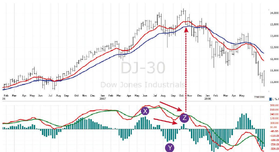
图23-4 道琼斯工业平均指数（DJIA）周线图，26日和13日指数移动平均线，12-26-9MACD线和柱状图
